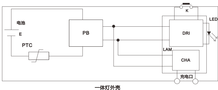
图 2 KL2.5LM(A)型矿灯工作原理
