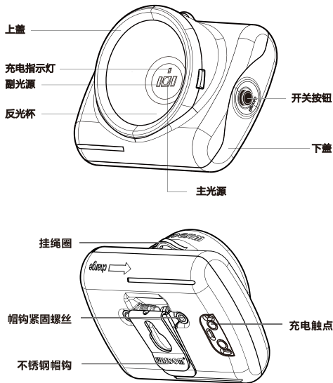
图 1 KL2.5LM(A)型矿灯结构
